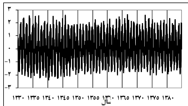
شکل ۸) سری زمانی مقادیر شاخص شدت پرفشار سیری در تراز ۱۰۰۰ هکتوپاسکال
