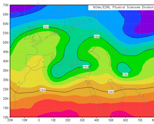
شکل ۱۲ E: دما تراز ۵۰۰ (۲۳ فوریه ۱۹۹۱)
