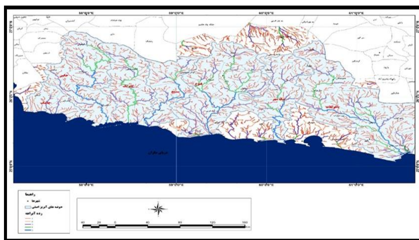
شکل ۲- رده آبراهه ها در حوضه های زهکشی منطقه بر اساس روش استرال
