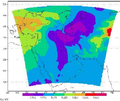
شکل ۸) نقشه فشار سطح دریا، خروجی مدل WRF (قلمرو اول در خاور میانه) در روز ۱۸ نوامبر ۲۰۰۱ (۲۷ آبان ۱۳۸۰)
