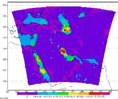
شکل ۱۰) نقشه جریان رطوبت سطحی روبه بالا (کیلوگرم بر مترمربع در ثانیه)، خروجی مدل WRF (قلمرو اول در خاور میانه) در روز ۱۸ نوامبر ۲۰۰۱ (۲۷ آبان ۱۳۸۰)
