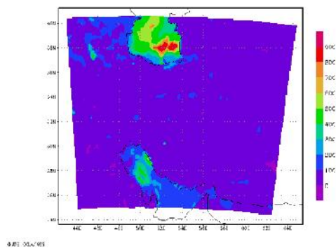
شکل ۶۷) نقشه گرمای نهان منطقه (وات بر متر مربع)، خروجی مدل WRF (قلمرو دوم در ایران) در روز ۲۲ اکتبر ۲۰۰۲ (۳۰ مهر ۱۳۸۱)
