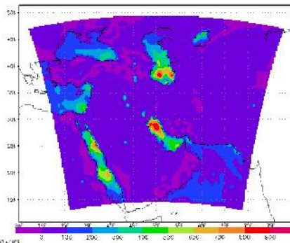
شکل ۱۲) نقشه گرمای نهان منطقه (وات بر متر مربع)، خروجی مدل WRF (قلمرو اول در خاور میانه) در روز ۱۸ نوامبر ۲۰۰۱ (۲۷ آبان ۱۳۸۰)
