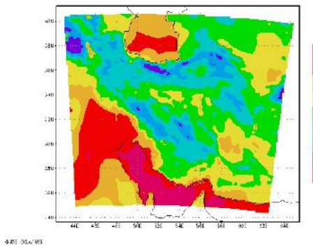
شکل ۲۸) نقشه دمای سطح دریا، خروجی مدل WRF (قلمرو دوم در ایران) در روز ۱۱ اکتبر ۲۰۰۰ (۱۰ مهر ۱۳۷۹)
