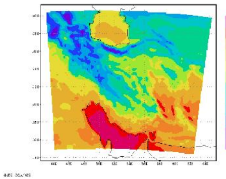
شکل ۳۰) نقشه دمای ۲ متری هوا، خروجی مدل WRF (قلمرو دوم در ایران) در روز ۱۱ اکتبر ۲۰۰۰ (۱۰ مهر ۱۳۷۹)
