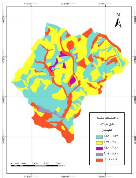
شکل ۳) لایه خاک‌شناسی حوضه آبخیز کن
