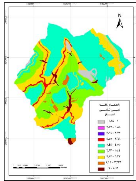
شکل ۲) لایه زمین‌شناسی حوضه آبخیز کن
