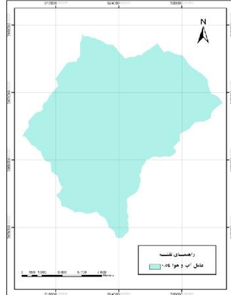
شکل ۶) لایه آب و هوای حوضه آبخیز کن
