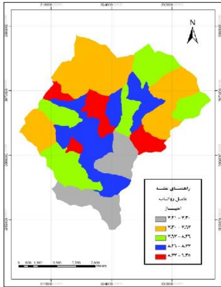
شکل ۵) لایه رواناب حوضه آبخیز کن
