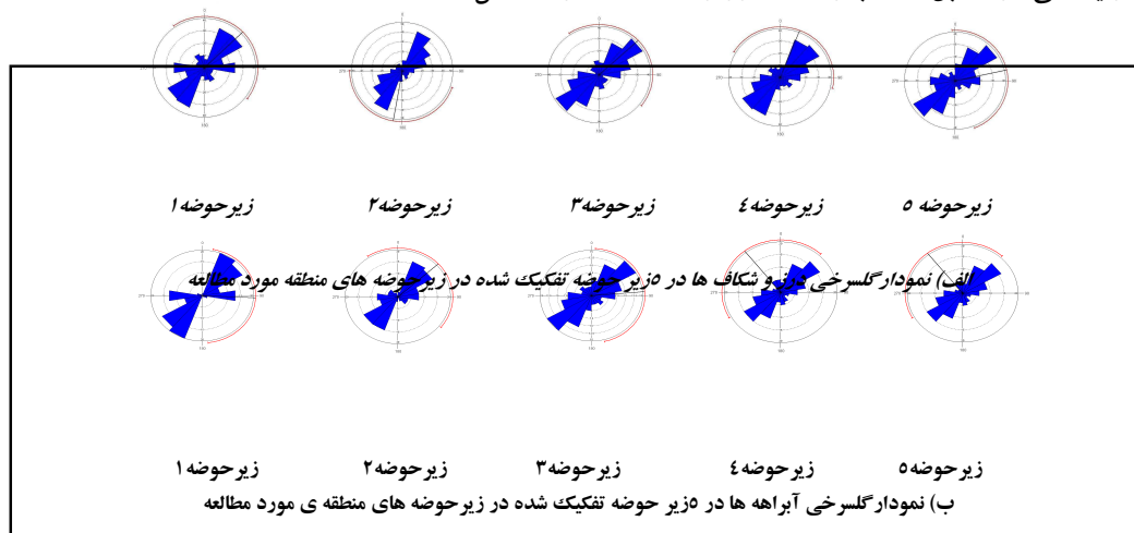
شکل ۱۰) نمودار گل‌سرخي آبراهه‌ها و درز و شکاف‌ها حوضه مورد مطالعه
