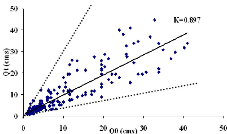
شکل (۲) پراکندگی نقاط در داده‌های دبی جریان در روش همبستگی منحنی افت اصلی
