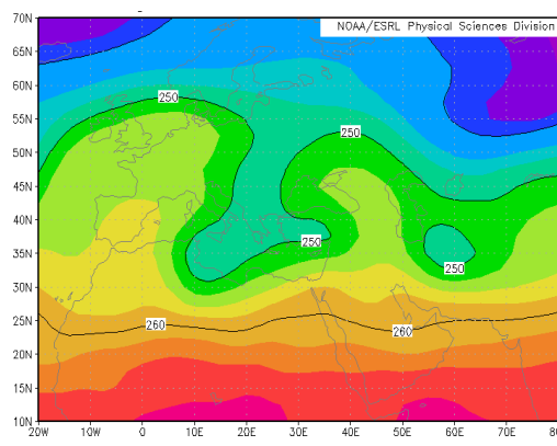
شکل ۱۲ E: دما تراز ۵۰۰ (۲۳ فوریه ۱۹۹۱)
