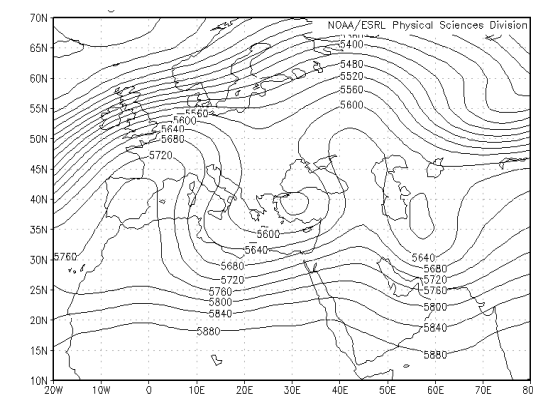
شکل ۱۲ F: ارتفاع تراز ۵۰۰ (۲۳ فوریه ۱۹۹۱)
