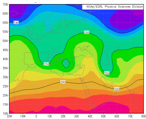
شکل ۱۲ C: دما تراز ۵۰۰ (۲۲ فوریه ۱۹۹۱)
