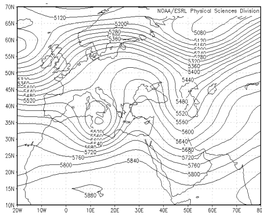
شکل ۱۲ B: ارتفاع تراز ۵۰۰ (21 فوریه ۱۹۹۱)
