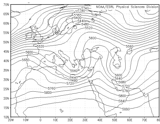
شکل ۱۲ D: ارتفاع تراز ۵۰۰ (۲۲ فوریه ۱۹۹۱)
