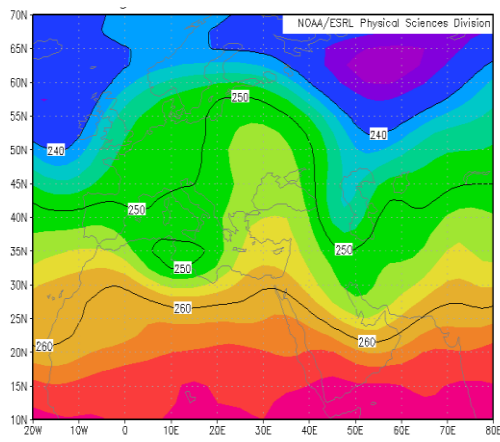
شکل ۱۲ A: دما تراز ۵۰۰ (۲۱ فوریه ۱۹۹۱)
