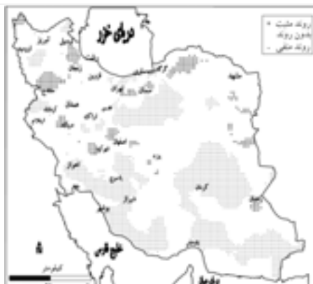
نگاره ۸) روند تعداد روزهای فرین سرد برج خرداد
