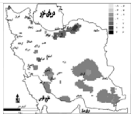
نگاره ۲۱) شیب روند برج آذر
