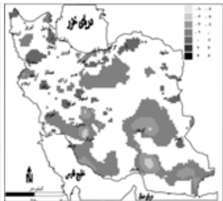
نگاره ۹) شیب روند برج خرداد
