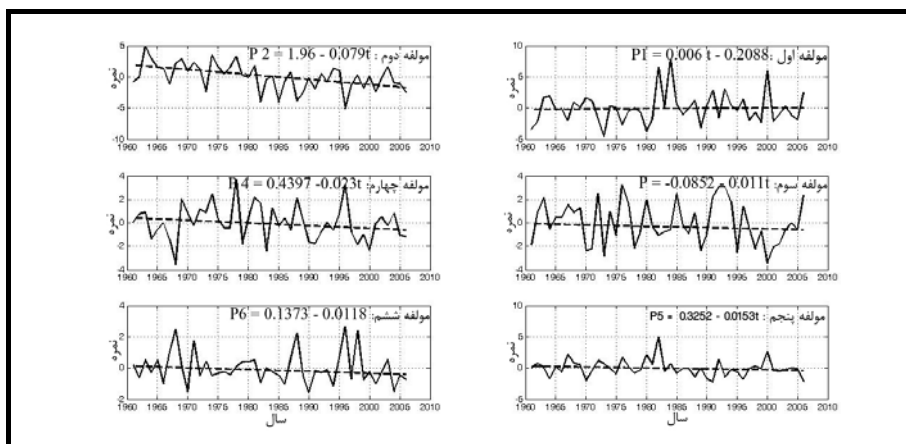
شکل ۱: تغییرات زمانی و روند شش مؤلفه مبنای نمایه‌های فرین بارش زنگان برای دوره آماری
