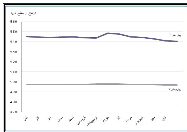
شکل ۶- مقایسه گراف‌های ماهانه پیژومترهای شماره ۲ و ۷
