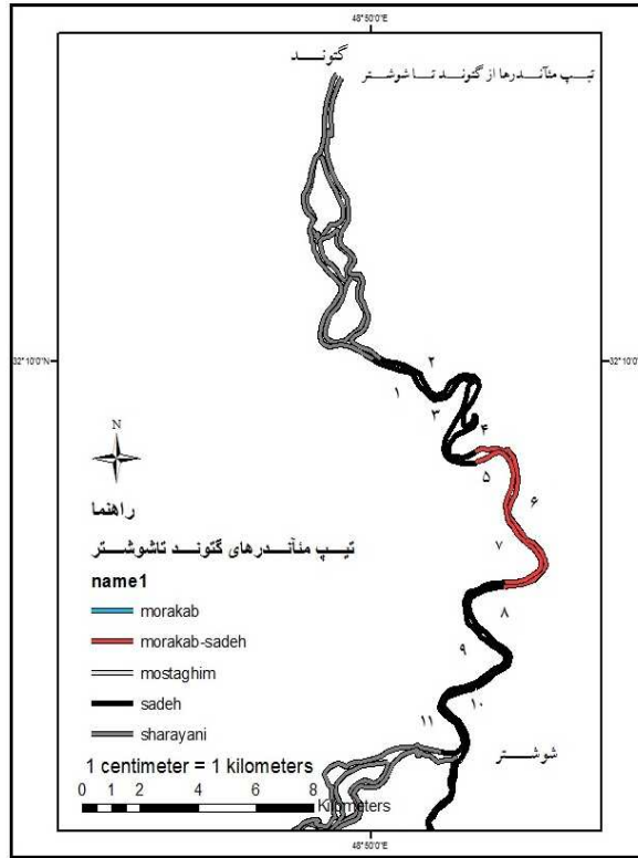
شکل ۳) نوع پیچان رودهای کارون از گتوند تا شوستر
