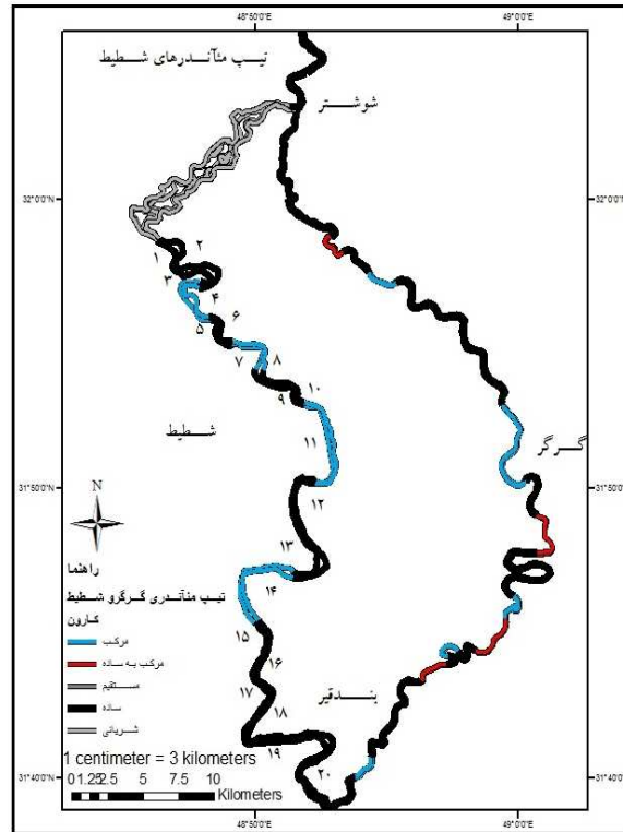
شکل ۴) نوع پیچان رودهای کارون از شوستر تا بند قیر (شطیط)
