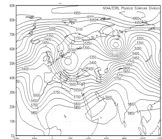
شکل ۱۳) نقشه تراز ۵۰۰ میلی بار روز ۲۰ / ۱۱ / ۸۴ ساعت ۱۲ زلو
