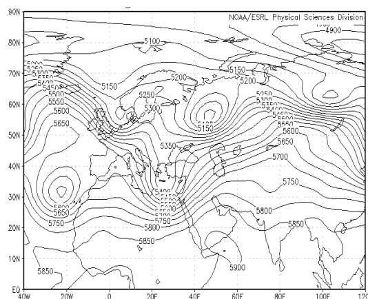
شکل ۹) نقشه تراز ۵۰۰ میلی بار روز ۲۰ / ۱۱ / ۸۴ ساعت ۱۲ زلو
