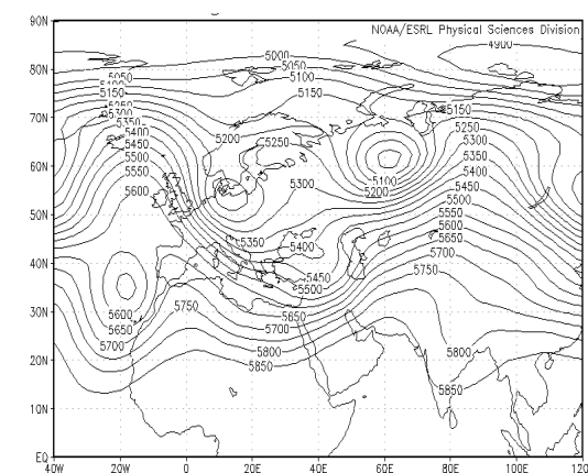
شکل ۱۱) نقشه تراز ۵۰۰ میلی بار روز ۲۰ / ۱۱ / ۸۴ ساعت ۱۲ زلو
