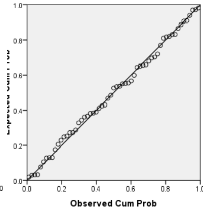
شکل ۱) پراکنش توزیع باقی مانده‌ها برای بارش خرم آباد
