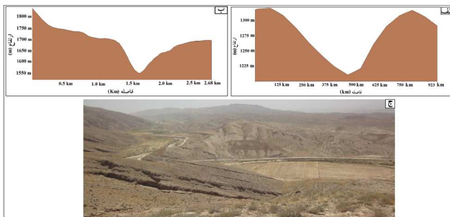
شکل ۱۰) نمایی از دره‌های منطقه: الف) دره ۷ شکل مربوط به پهنه شماره ۲، ب) دره ۷ شکل مربوط به پهنه شماره ۶، ج) دره U شکل مربوط به پهنه شماره ۲۰
