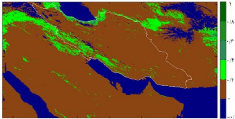
شکل ۸- میانگین پوشش گیاهی فصل بسیار تنک در بازه‌ی ۴ آذر تا ۷ اسفند
