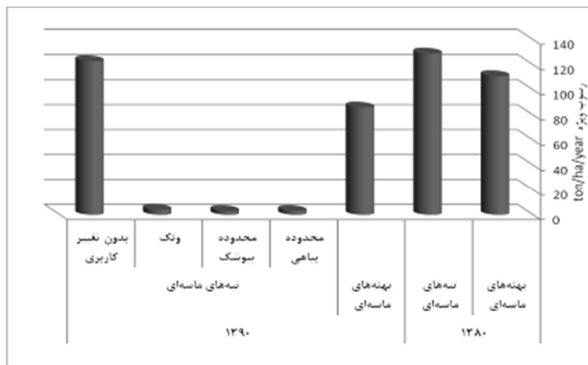
شکل ۵) رسوب ویژه بادی در دو مقطع زمانی ۱۳۸۰ و ۱۳۹۰
