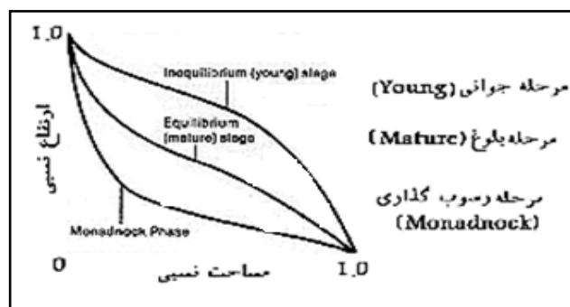
شکل ۵- سه حالت از منحنی هیپسومتری
