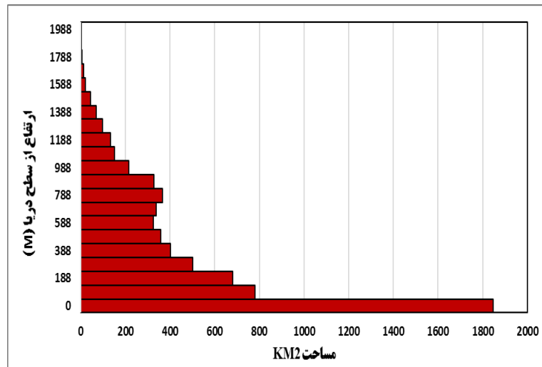
شکل ۸- منحنی آلتیمتری کل حوضه زهكشی منطقه مطالعاتی
