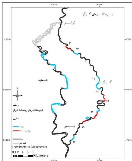
شکل ۵) نوع پیچان رودها از بازه شوشتر تا بند قیر (رودخانه گسرگر)
