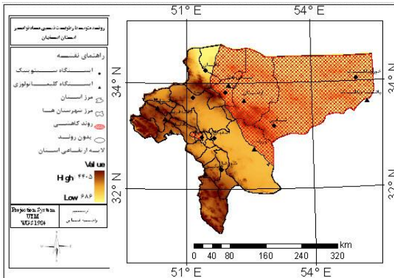
شکل ۱۳ - پهنه‌بندی روند متوسط رطوبت نسبی ماه نوامبر
