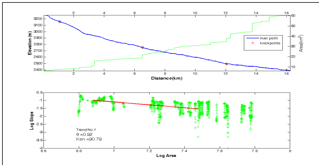
شکل ۸- نمودارهای نیمرخ طولی و نیمرخ توزیع شیب و رگرسیون لگاریتمی آبراهه اصلی حوضه تاجبار
